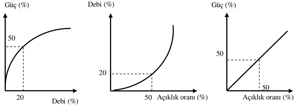
Şekil 2.6 Isı yükü ile vana açıklığı arasında oransal değişim elde edilmesi
